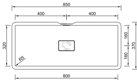
FMP-80-32
