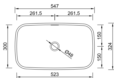
FCU-52-30
