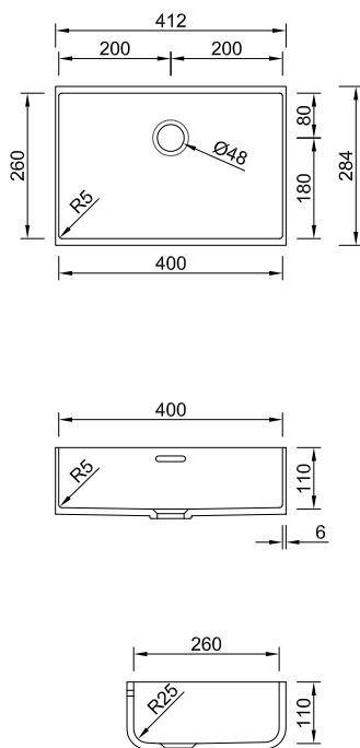
FP-40-26
