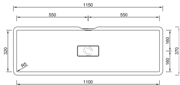
FMP-110-32
