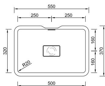
FMS2-50-32
