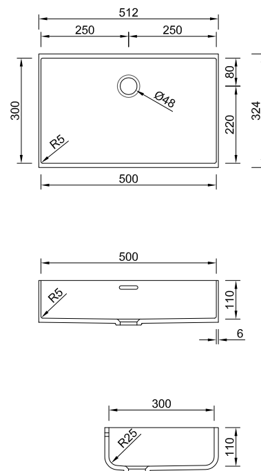
FP-50-30
