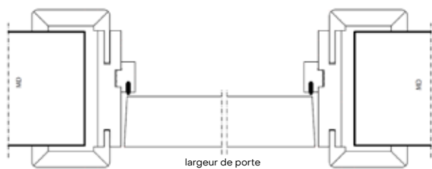
WoodFlex Vantail en retrait par rapport aux chambranles
