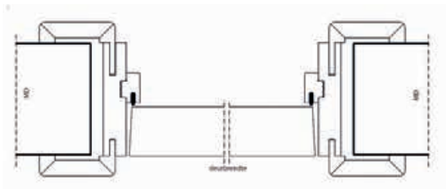
Horizontale doorsnede WoodFlex kozijn Section horizontale huisserie WoodFlex
