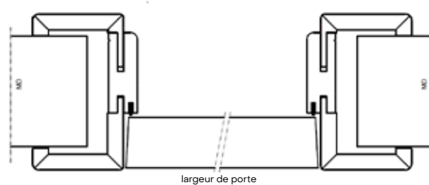
WoodFlex Style Vantail affleurant avec les chambranles (en onglet)
