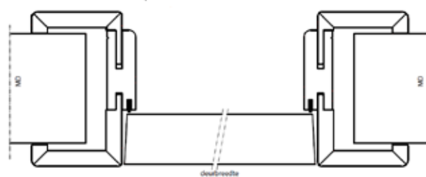
WoodFlex Style Deurblad in gelijk vlak met deurlijsten (in verstek)
