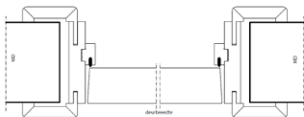
Horizontale doorsnede WoodFlex kozijn
