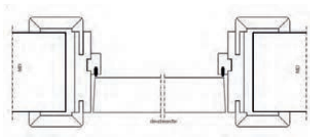
Horizontale doorsnede WoodFlex kozijn
