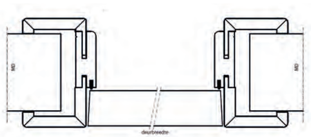
Horizontale doorsnede WoodFlex Style kozijn
